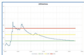
Lokální výstražný systém – hladinoměr u Surých při horním obchodu – průběh hladin
